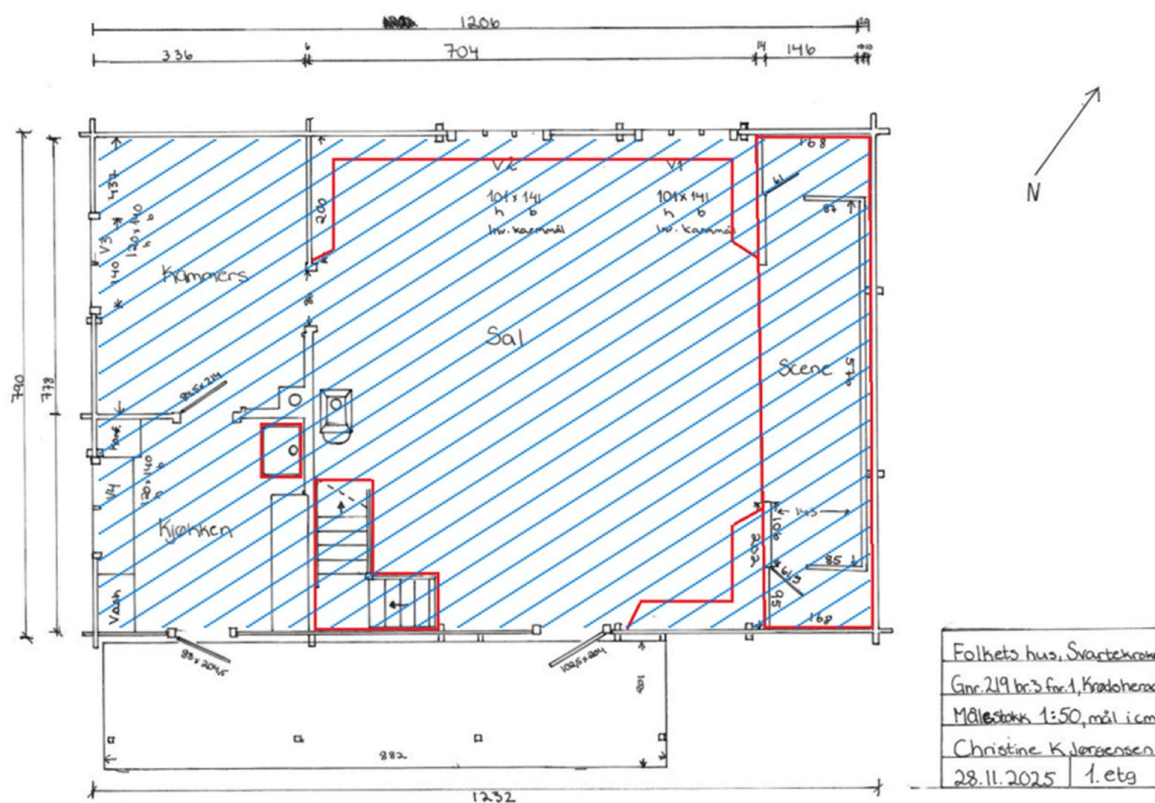
Plantegning, 1. etasje. Interiørfredningen er markert med blå skravur.
